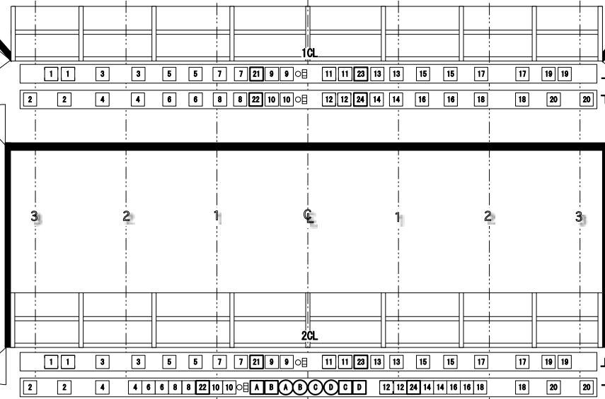
世田谷区庁舎F.O.H 7F回路図
